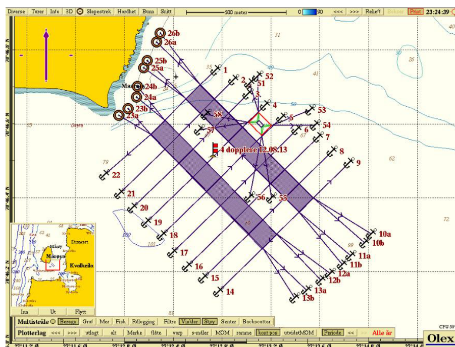
Vedlegg 6.1.3 Anlegg med fortøyning. Posisjon for strømmåling avmerket. Bunntopografi fra sjøkart (hentet fra søknaden)
